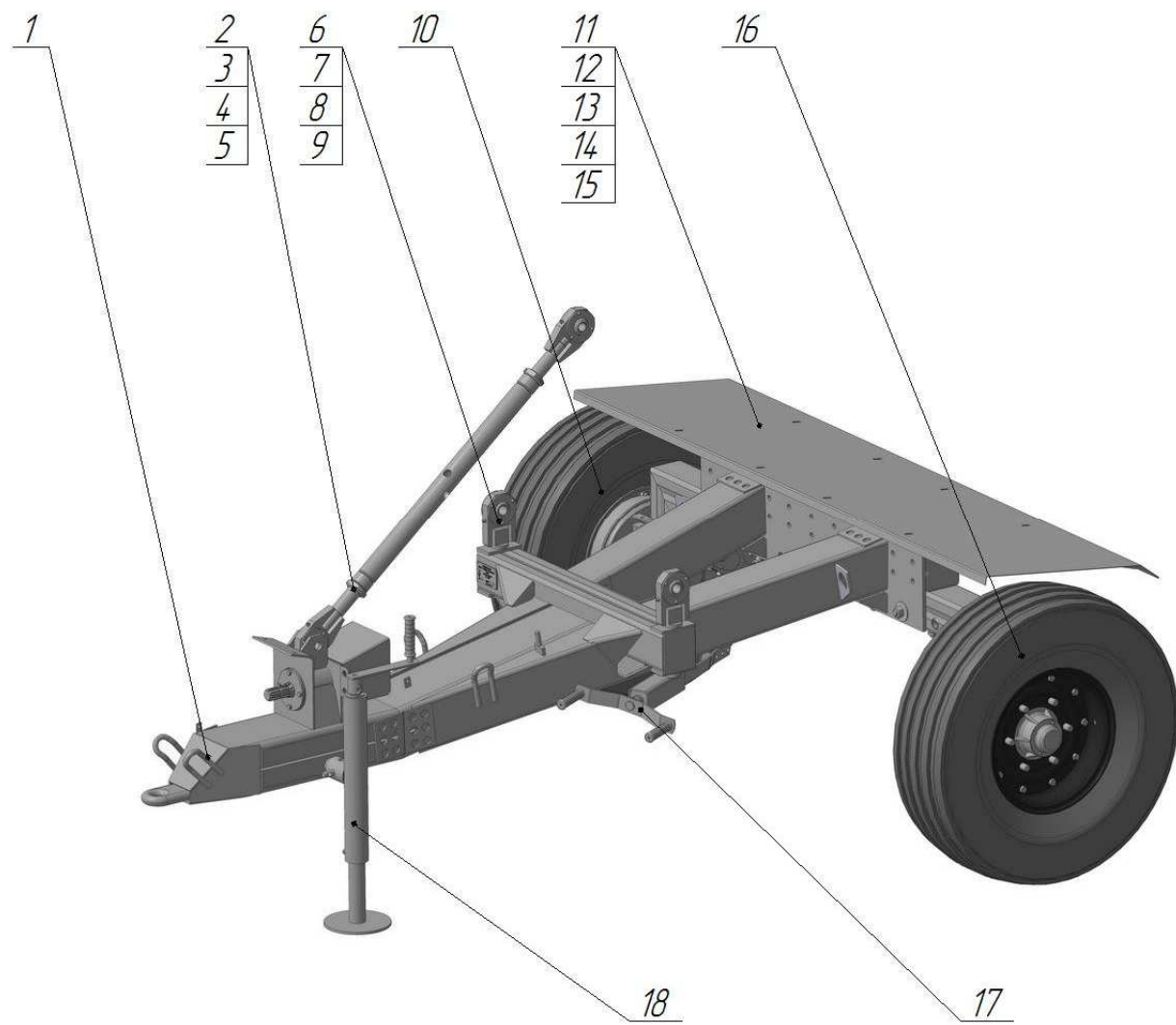
Рисунок 13 – Шасси технологическое
