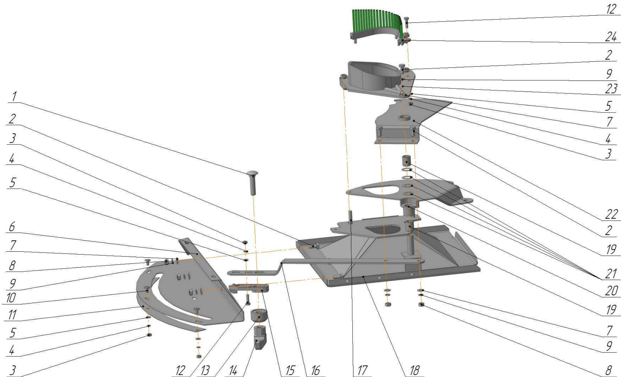
Рисунок 8 – Узел дозирующий
