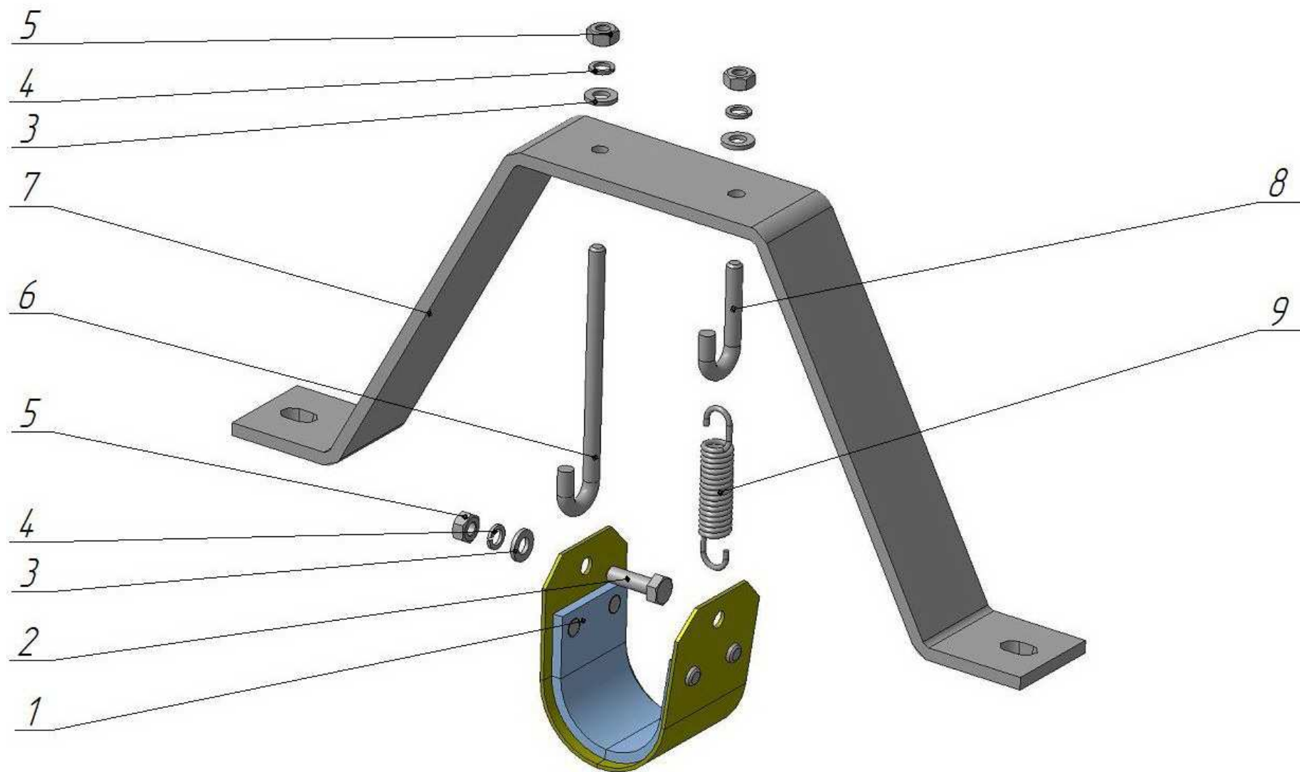
Рисунок 7 – Тормоз
