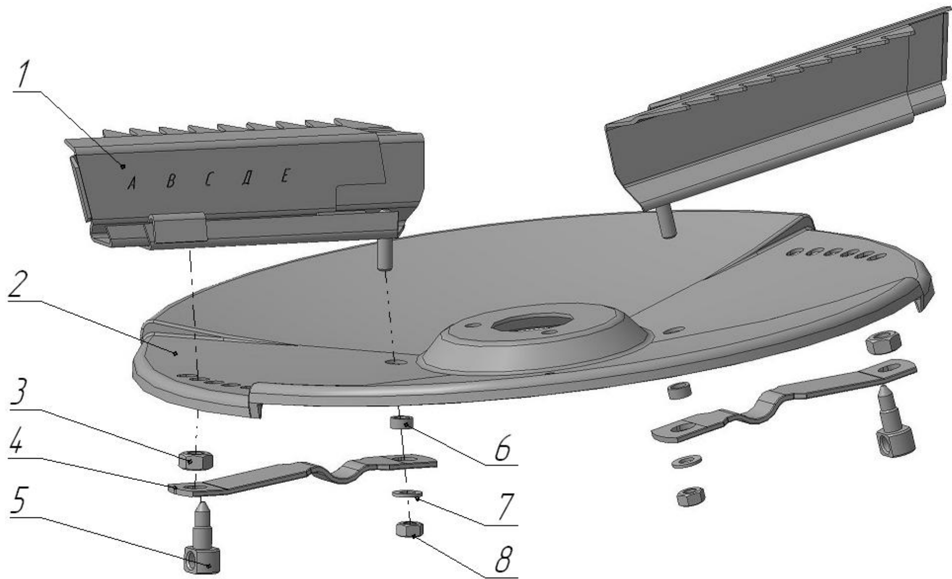
Рисунок 6 – Метатель
